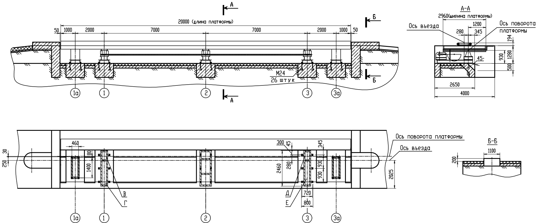
Нагрузка на опоры автомобилеразгрузчика АВС-60
