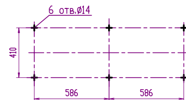
План расположения фундаментных болтов Башмака нории
